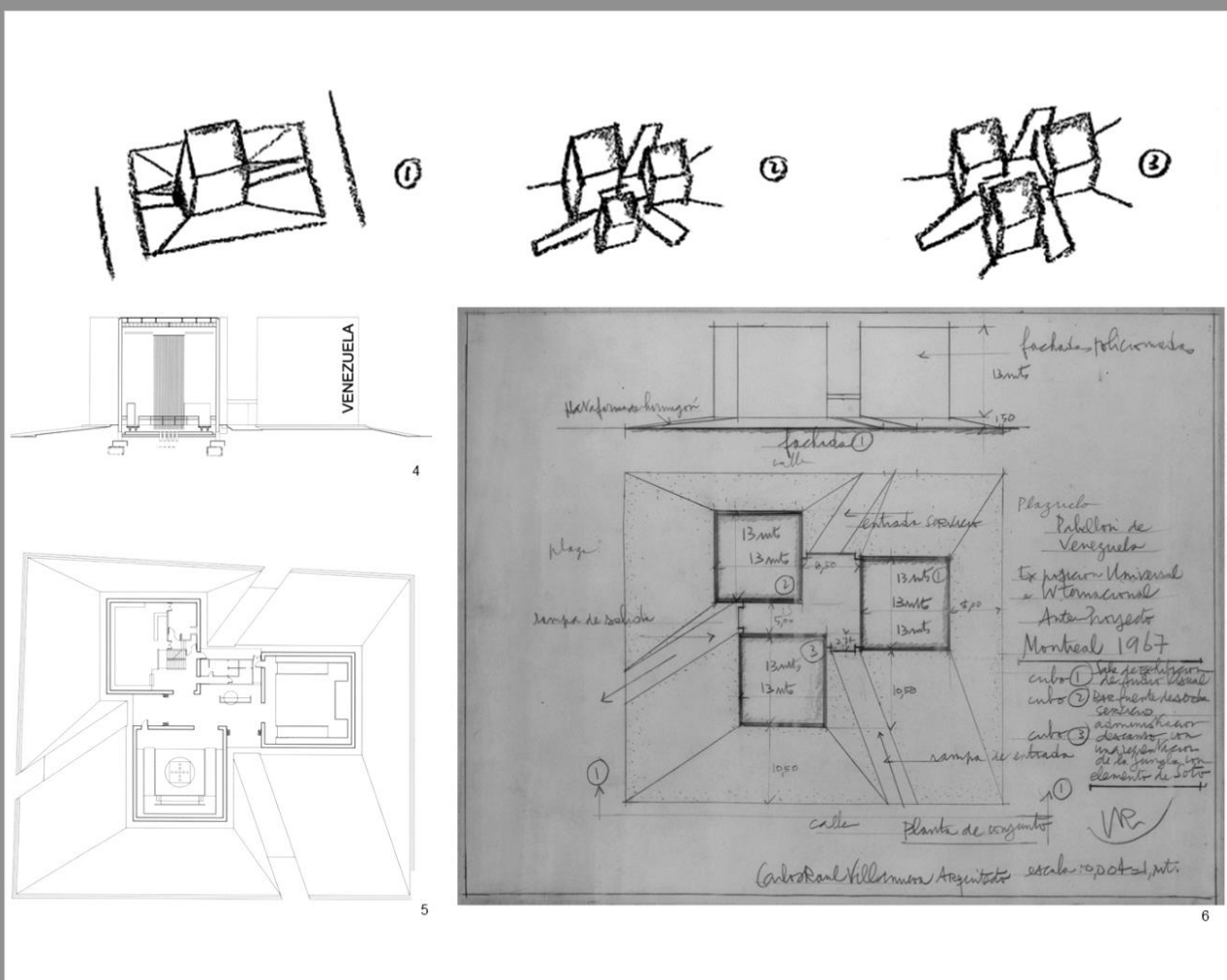
Concepto del "Pabellón de Venezuela" para la Exposición de Montreal, 1967, en Canadá. 1, 2, y 3 Croquis de Evolución de idea, 4 Sección y Alzado, 5 Planta baja, 6 Dibujo del anteproyecto, 7 Detalle interior del cubo con la instalación de Soto. Concepto del Proyecto. En: VILLANUEVA, Paulina y PINTO, Maciá (2000) Carlos Raúl Villanueva. Serie Maestros Latinoamericanos de la Arquitectura. Madrid. Tanais Ediciones, S.A. p.140
